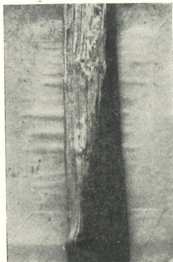
Fig. 1. — Secțiune longitudinală printr-o porțiune de trunchi injectată cu colorant.
