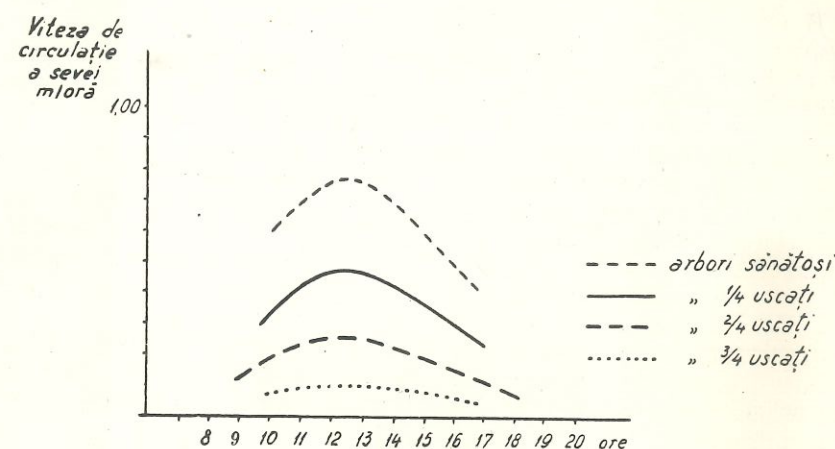
Fig. 3. — Circulația sevei la arbori în diferite faze de uscare în timpul unei zile.
