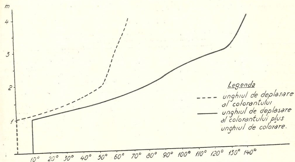
Fig. 7. — Mișcarea laterală a colorantului la arborele nr. 7.
