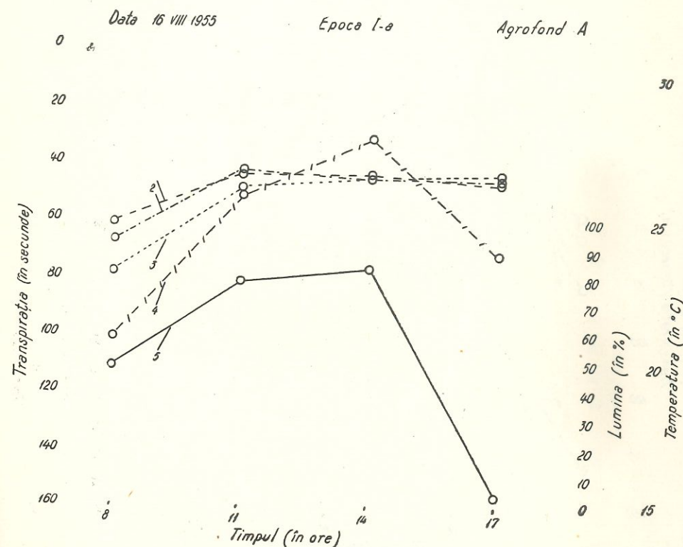
Fig. 3. — Mersul transpirației în timpul zilei la porumbul I.C.A.R. 54 (îngrășat). 1, Varianta 70/50 cm; 2, varianta 75/75 cm; 3, varianta 80/80 cm; 4, intensitatea luminii; 5, temperatura aerului.
