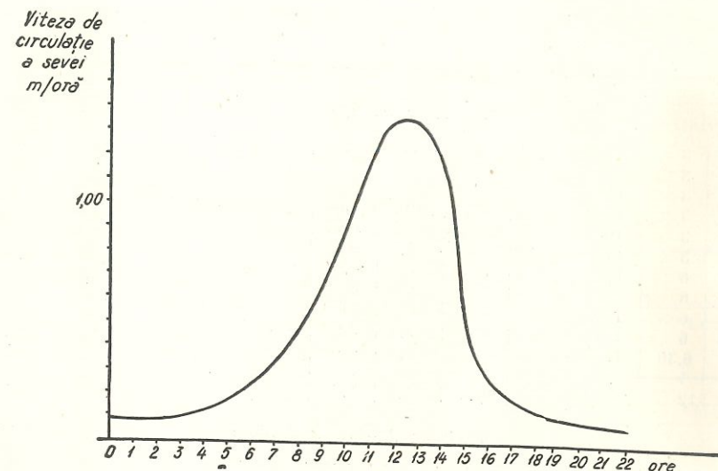
Fig. 2. — Variația vitezei de circulație a sevei la pinul negru în decursul unei zile senine de august.
